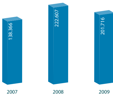
Emisiones directas de CO 2 y CH 4 (t CO 2 eq)
